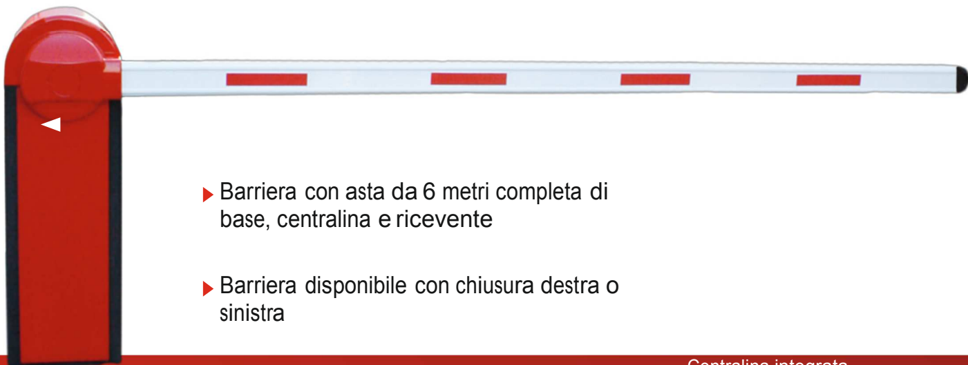
Barriera ASB-6010 con chiusura a destra FM 434,42 MHz: codice 7628V001
