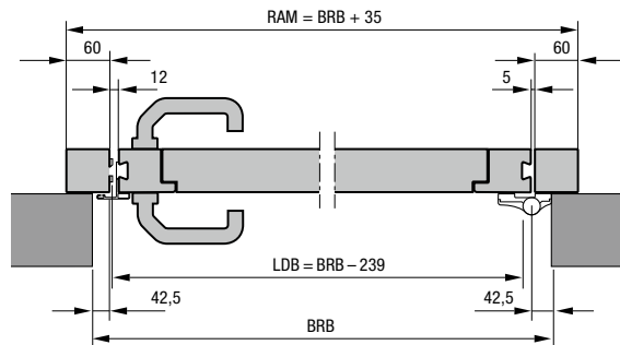
Sezione orizzontale
