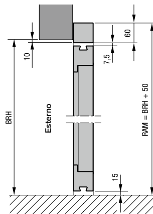
Sezione verticale
