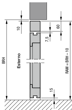
Sezione verticale
